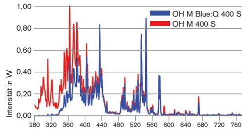
Vergleich der spektralen Bestrahlungsstärke „OH M 400 S“ und „OH M Blue:Q 400 S“
